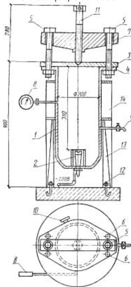
1 — корпус; 2 — нагревательные электроды; 3 — крышка; 4 — верхний фланец; 5 — бугельные болты; 6 — фланцевые болты; 7 — двухплечий бугель; 8 — электроконтактный манометр ЭКМ-1; 9 — кран для спуска пара и воздуха; 10 — предохранительный клапан; 11 — упорный винт; 12 — фундаментные болты; 13 — опоры; 14 — защитный кожух автоклава Черт. 4
