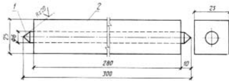
1 — стержень из нержавеющей стали; 2 — изолирующая оправа (дуб с последующим покрытием наружной поверхности лаком) Черт. 3
