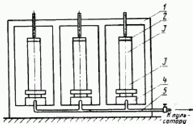
1—рама машины; 2—вертикальный винт с оголовником; 3—образец; 4—гидрозомкрат; 5—масляный привод.
